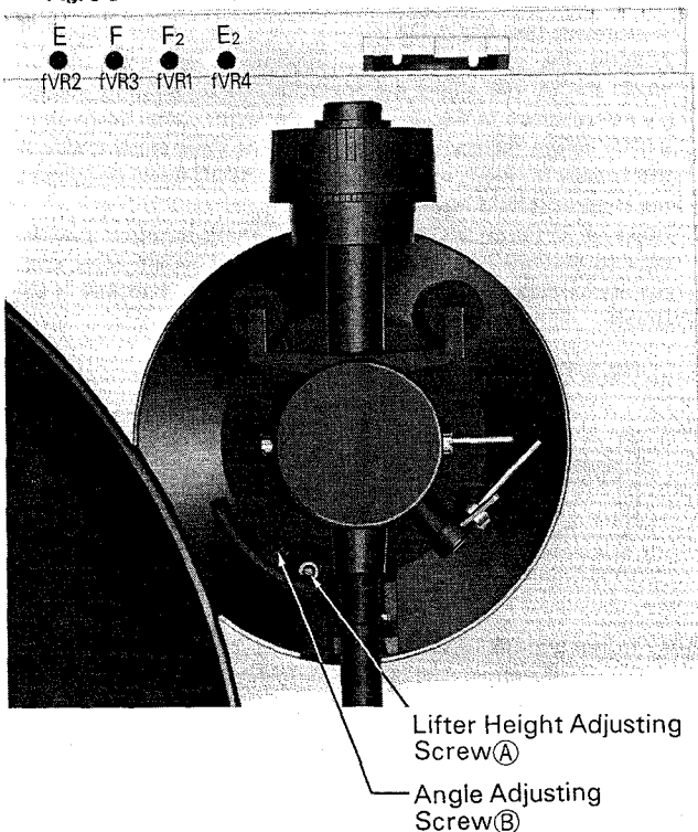
Fig. 3-5
