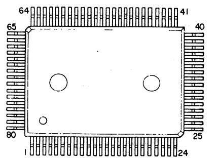
CXD2500Q
