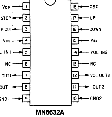
MN6632A SM5840
