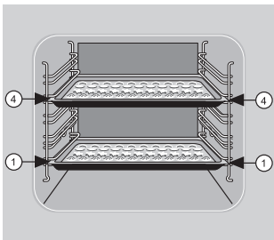
2 Backbleche: Einsatzebenen 1 und 4
