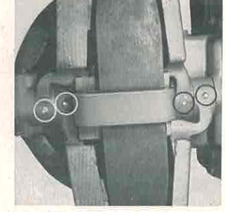
14 Gliederbolzen 4 Schmierstellen
