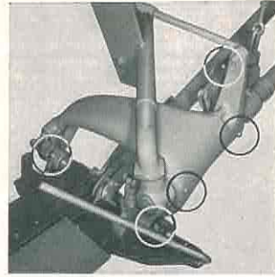
2 Scharnierbrücke 5 Schmierstellen
