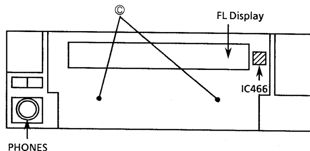
Fig 4. Front P.C. Board(ENC-071-10)
